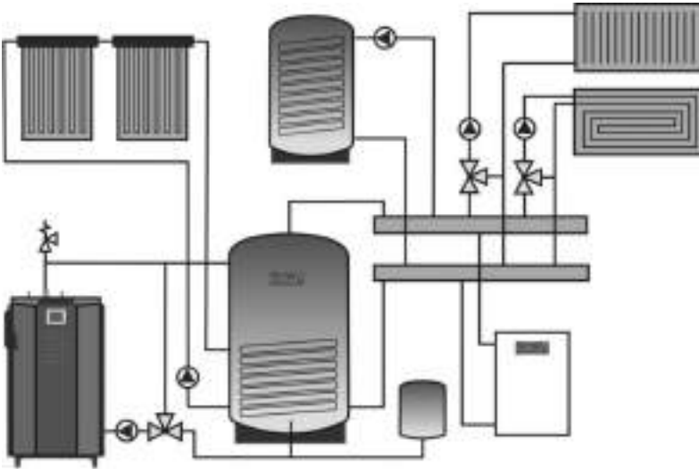
Schéma č. 3 – Zapojení zplyňovacího kotle s akumulční nádrží s výměníkem pro solární ohřev, nádrží na TUV, solárními panely, směšovacími topnými okruhy (radiátorovým a podlahovým) a automatickým kotlem (např. plynovým).
