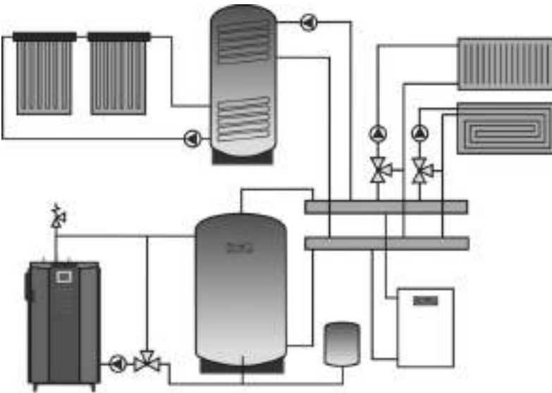
Schéma č. 4 – Zapojení zplyňovacího kotle s akumulční nádrží, nádrží na TUV s výměníkem pro solární ohřev, solárními panely, směšovacími topnými okruhy (radiátorovým a podlahovým) a automatickým kotlem (např. plynovým).
